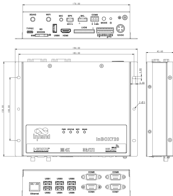
InBOX720产品尺寸图
