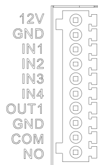
10脚接线端子接口图
